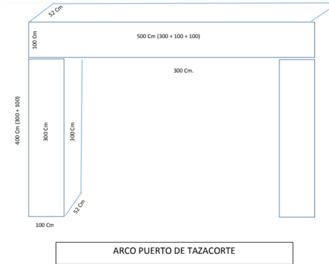
Ilustración 2. Croquis vinilado truss Lote 2
