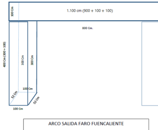
Ilustración 2. Croquis vinilado truss Lote 2
